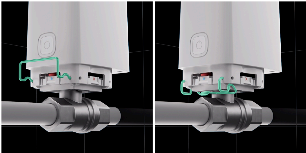
Стандартна монтажна скоба
